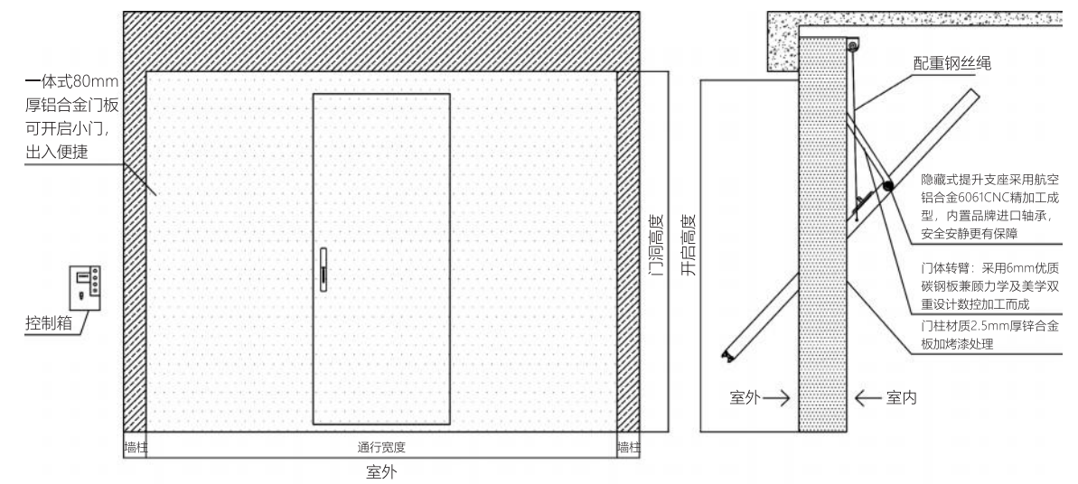
整板无轨上升车库门臻品系列相关参数
